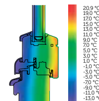
PRŮBĚH IZOTERM
