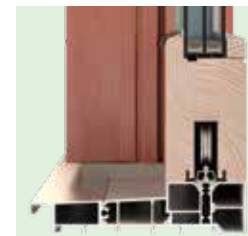
PRÁH S POJEZDOVÝM KŘÍDLEM
