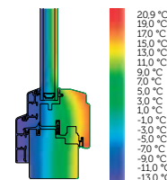
PRŮBĚH IZOTERM
