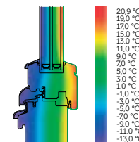
PRŮBĚH IZOTERM
