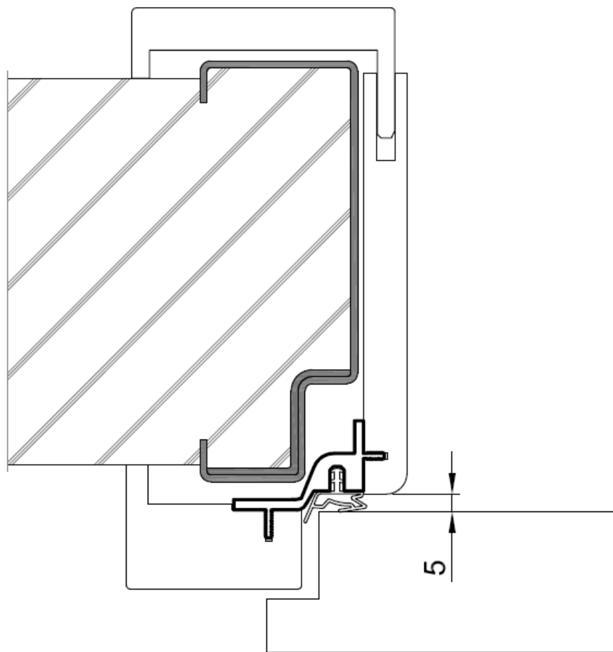
Původní provedení OKZ – těsnění vystupuje z ostění, mezera mezi křídlem a ostěním je cca 5 mm
