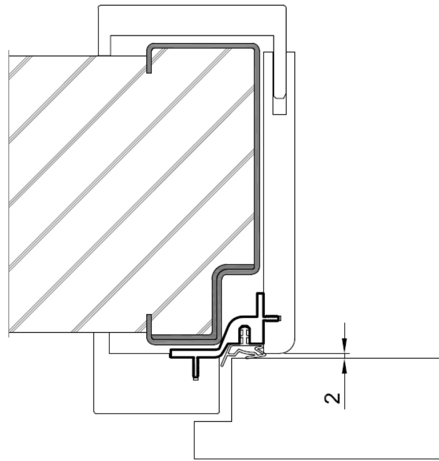
Nové provedení OKZ – profil s těsnění je zapuštěný do ostění, mezera mezi křídlem a ostěním se zmenšila na cca 2 mm
