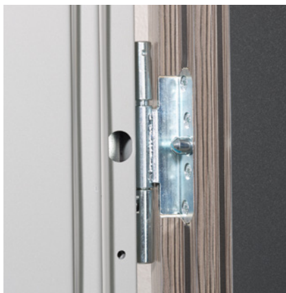
Třídílný zavěs s pasivním čepem
